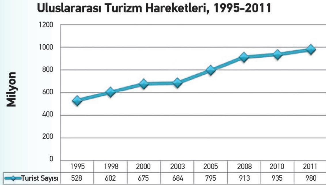
Uluslararası Turizm Hareketleri, 1995-2011
